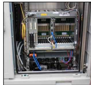
„Innenleben“ eines Multifunktionsgehäuses in Roßlau, Berliner Straße – Vectoring DSLAM 2510
